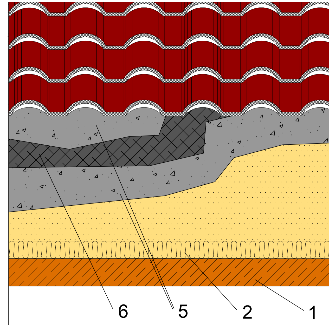
FALDÓN
