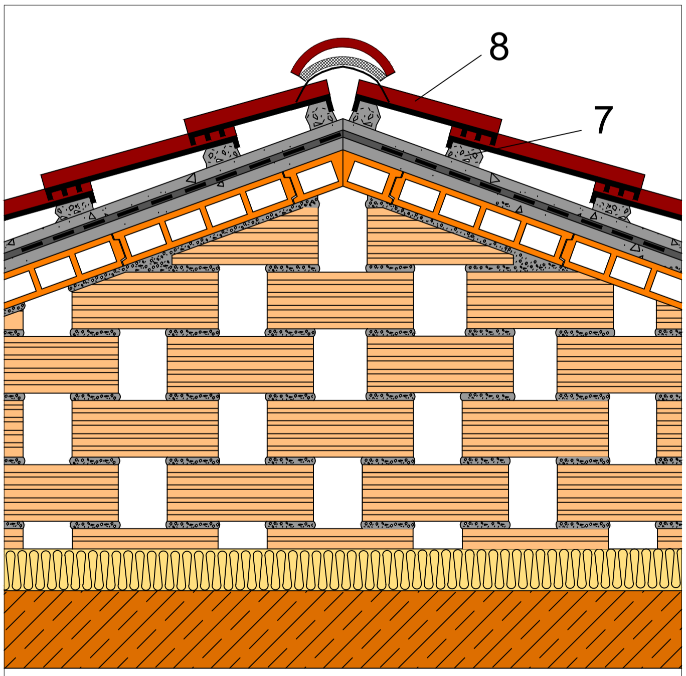
CUMBRERA
