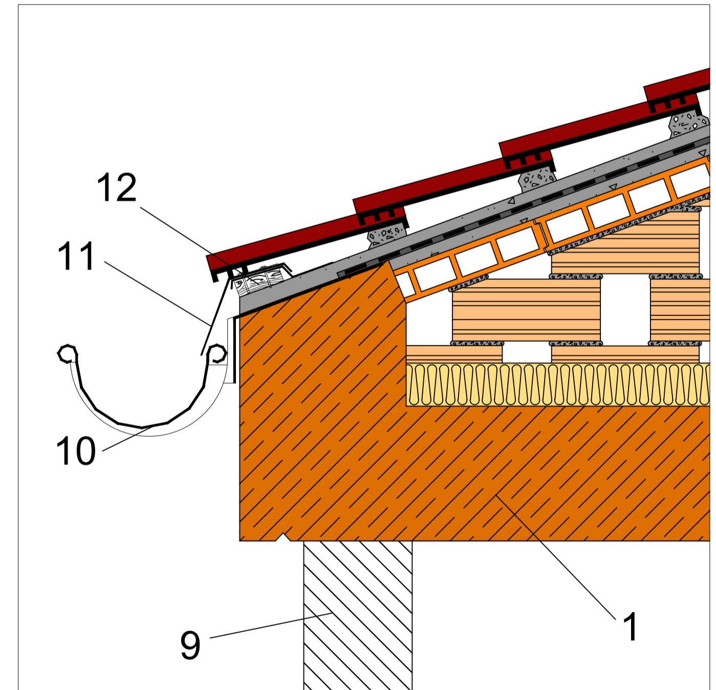
ALERO
