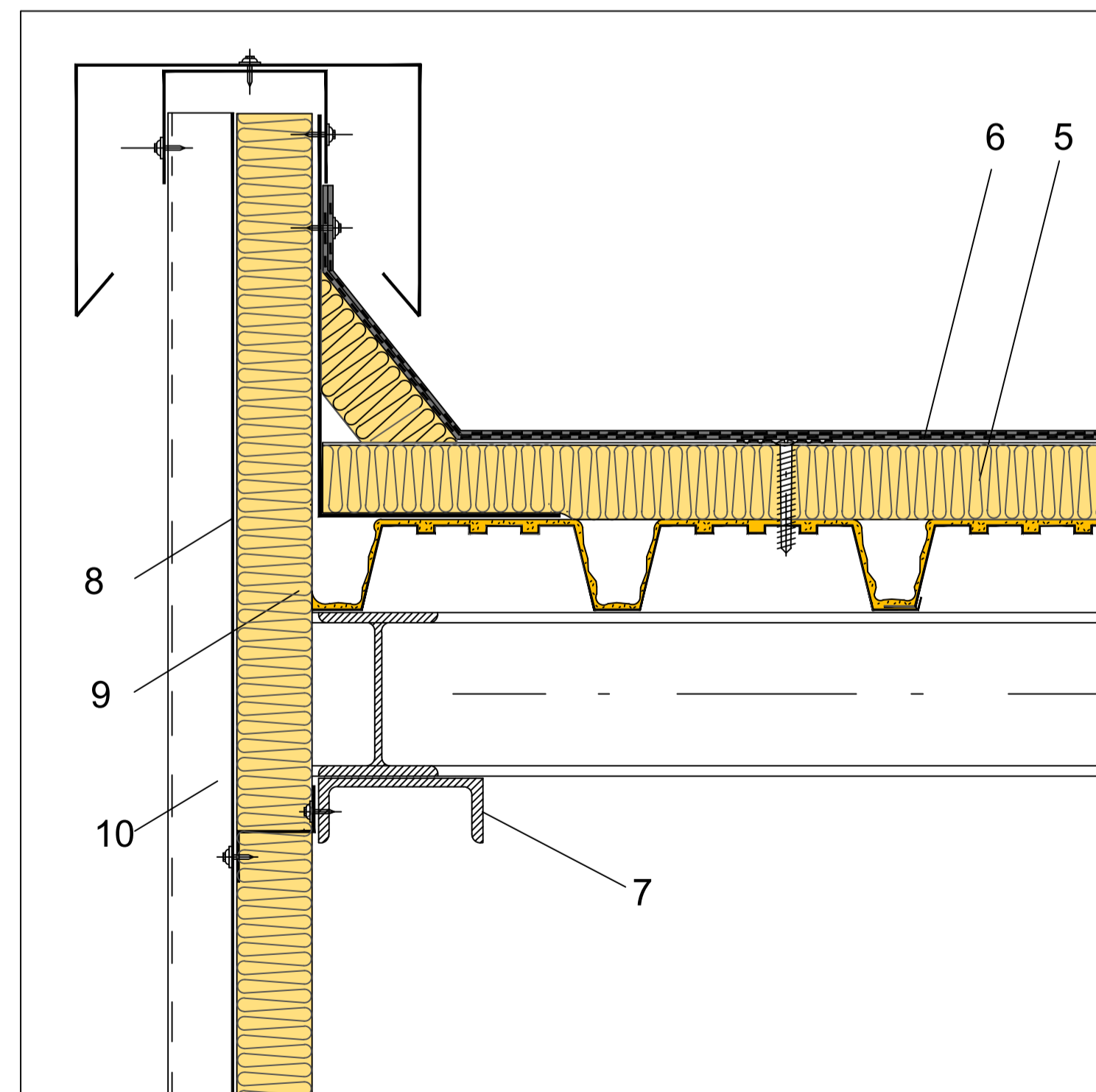
ENCUENTRO CON PARAMENTO VERTICAL
