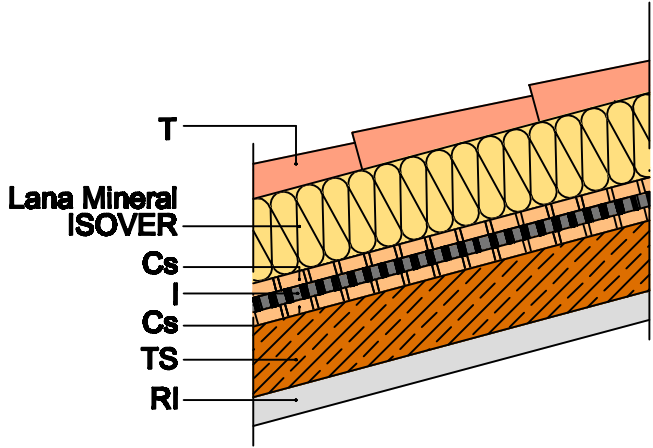
Cubierta invertida
