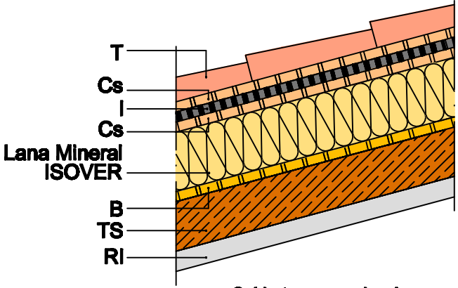
Cubierta convencional
