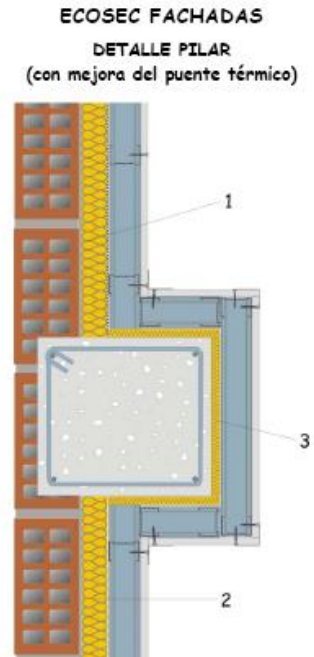
Fig. 10. Detalle de encuentro con pilar
